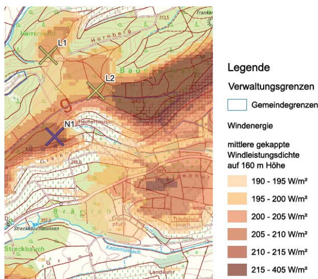
Abbildung 1: Auszug aus Karte mit Daten des Windatlases [Quelle: ZEAG]
